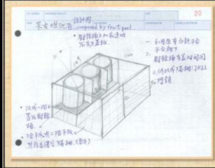
廚餘堆肥手繪圖
