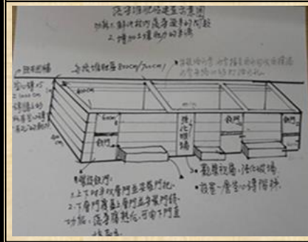
落葉堆肥手繪圖
