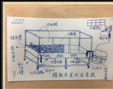
魚菜共生系統各項裝置手繪圖
